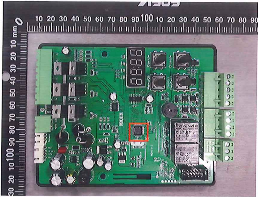
图 2 D158 主控板主芯片位置
