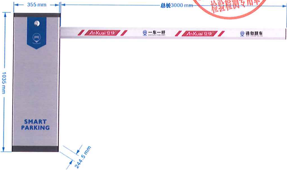
图 1 AK158-47-116-S580 型电动栏杆机配 G4 型 3.0m 直杆外形结构尺寸图
